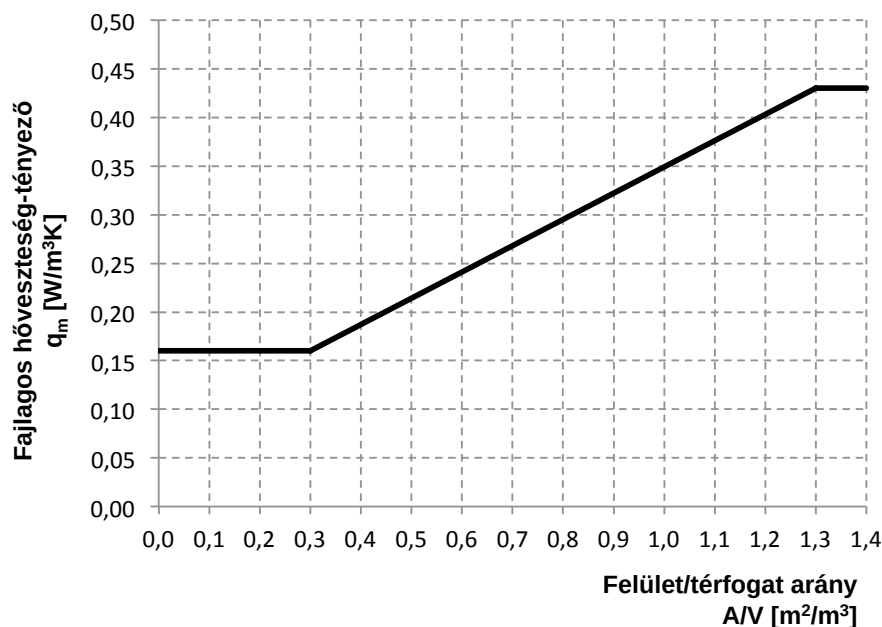
2.1 ábra. A fajlagos hővesztés-tényező követelményértéke
