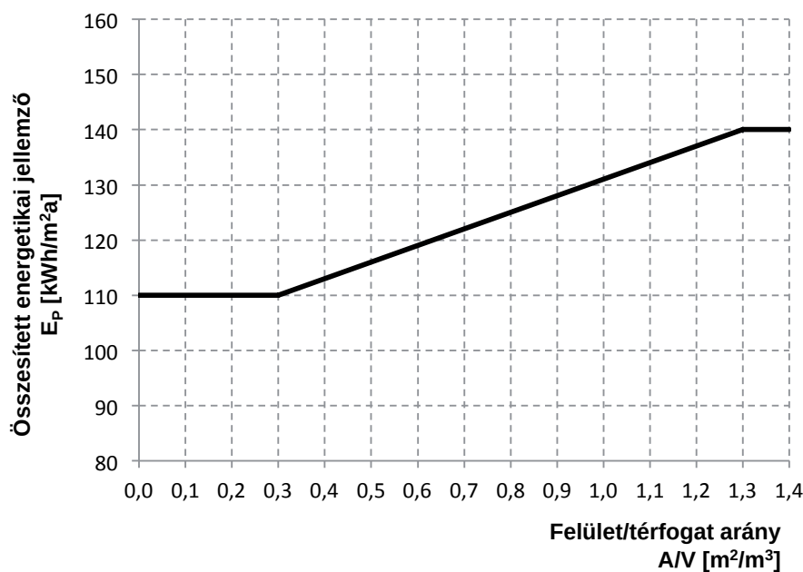
3.1. ábra: Lakó- és szállásjellegű épületek összesített energetikai jellemzőjének követelményértéke (nem tartalmazza a világítási energia igényt)
