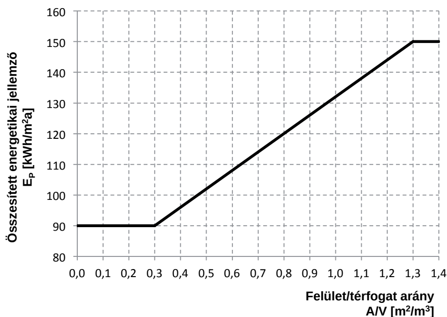
3.3 ábra: Oktatási épületek összesített energetikai jellemzőjének követelményértéke (világítási energia igényt is beleértve)
