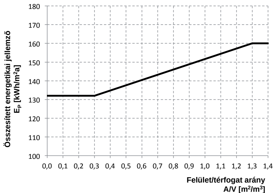
3.2. ábra. Irodaépületek összesített energetikai jellemzőjének követelményértéke (a világítási energia igényt is beleértve)
